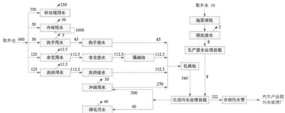
图 1 达祥公司现有项目水平衡图（ \text{m}^3/\text{d} ）
