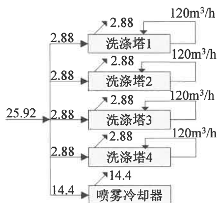
图 2 本技改项目水平衡图（ \text{m}^3/\text{d} ）
